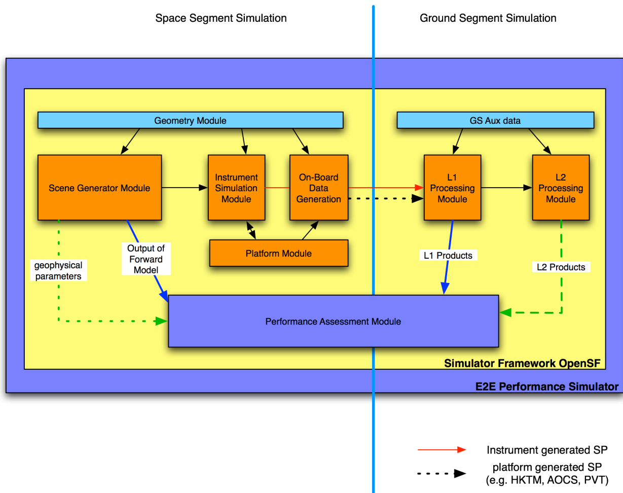
Fig. 3-1 E2E Performance Simulator
